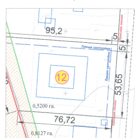
Генплан участка
