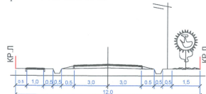
Поперечный профиль улицы промышленной зоны II-II
